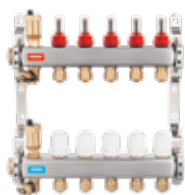
DISTRIBUITOARE-COLECTOARE DIN OȚEL INOXIDABIL 302
